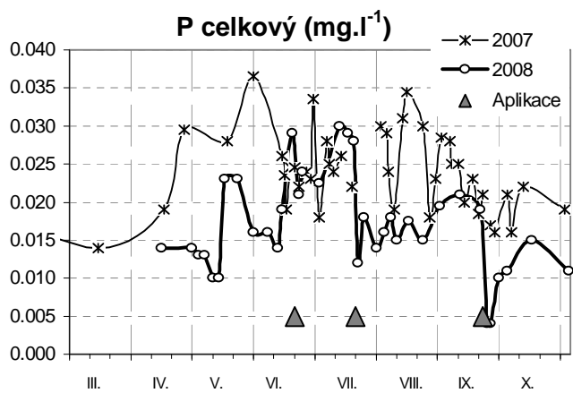
Obr.1 Sezónní průběh čtyř z nejdůležitějších ukazatelů kvality vody, porovnání druhého (2007) a třetího (2008) roku projektu. Trojúhelníčky jsou okamžiky aplikace PAXu v r. 2008. Na jaře za rozvoje parožnatků je vidět vysoká průhlednost, nízký obsah nerozpuštěných látek a nízká koncentrace P. Začátkem června, když parožnatky ustoupily, došlo ke zhoršení všech ukazatelů. Dobře je patrný pozitivní vliv aplikací Al koagulantu a úplná absence letního rozvoje sinicového vodního květu v r. 2008.
