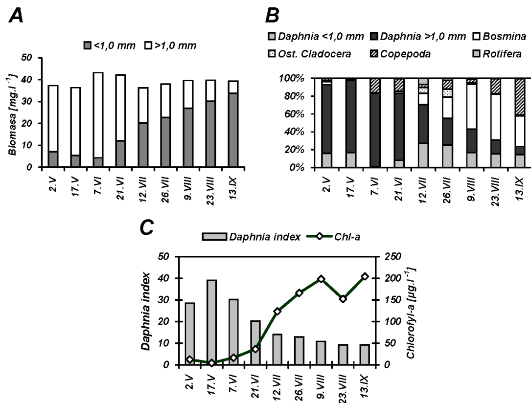
Obr.2 Sezónní průběhy celkové biomasy zooplanktonu (rozdělené na frakce <1,0 mm a >1,0 mm) (A), frekvencí (%) hlavních taxonomických skupin zooplanktonu (B) a Daphnia indexu a koncentrace chlorofylu-a (C) (rybník Humlena 5, 2005).
