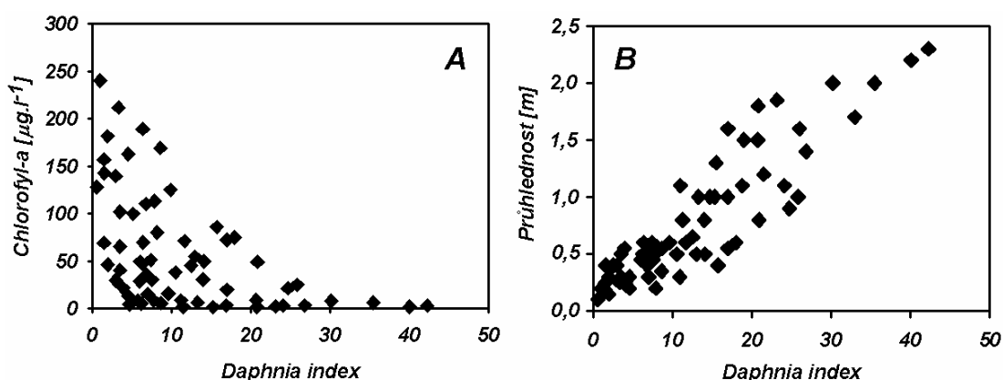
Obr.1 Vztah mezi Daphnia indexem a koncentrací chlorofylu-a (A) a Daphnia indexem a průhledností vody (B).
